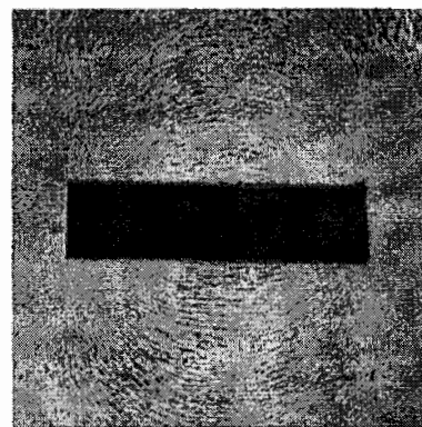
Hình 11. Ví dụ : từ phổ của một nam châm.
