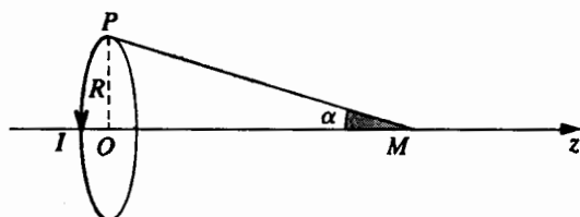
Hình 6. Vòng dây tròn.
