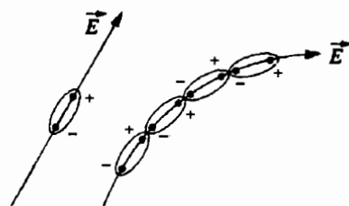
Hình 7. Cụ thể hóa một đường sức của trường.
