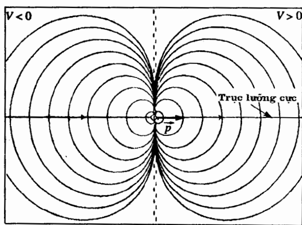
Hình 10. Đẳng thế của một lưỡng cực.
