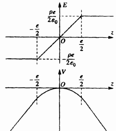
Hình 11. Trường E và thế V tạo ra bởi lớp phẳng vô hạn dày e và có mật độ điện khối đều \rho .
