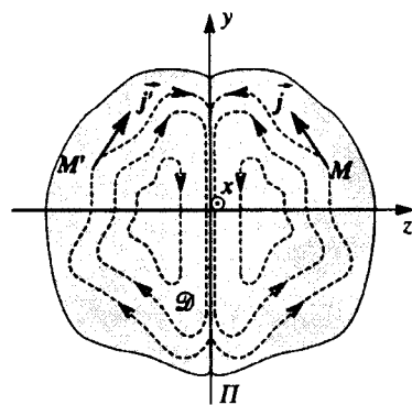
Hình 13. Đối xứng phẳng.
