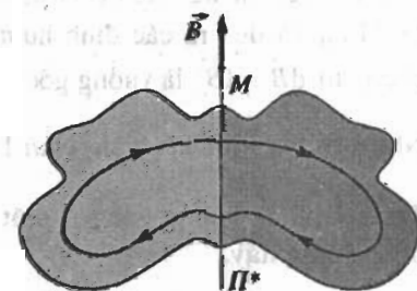
Hình 20a. Trường trên một mặt phẳng phản đối xứng.
