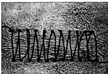
Hình 10. Ví dụ : Từ phổ của một ống dây (xôlênit - tập hợp các vòng dây)
