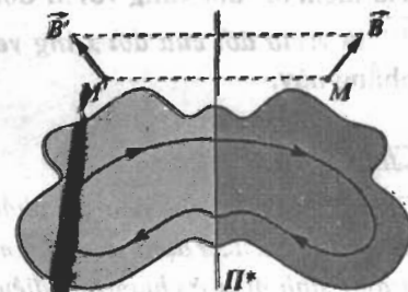
Hình 20b. Trường của hai điểm đối xứng.
